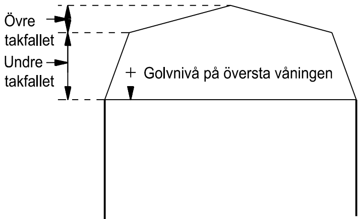
Principskiss över hur mansardtak beräknas.
